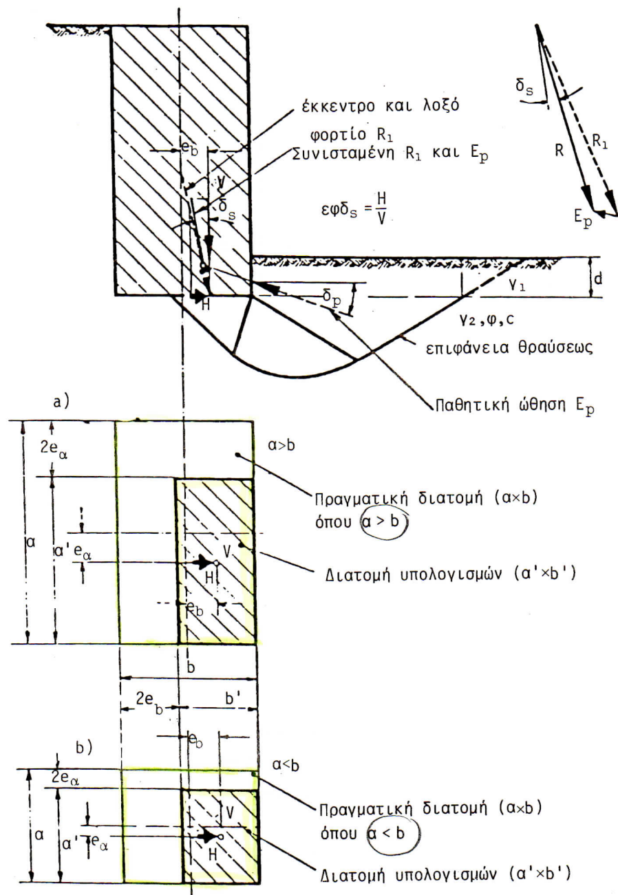
Σχήμα 2.21: Έκκεντρο και λοξό φορτίο παράλληλο προς τη μικρότερη πλευρά b , κατά DIN 4017, φύλλον 2.
