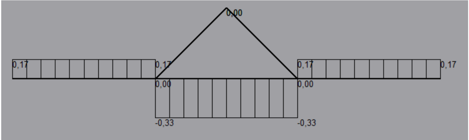
Διάγραμμα αξονικών
