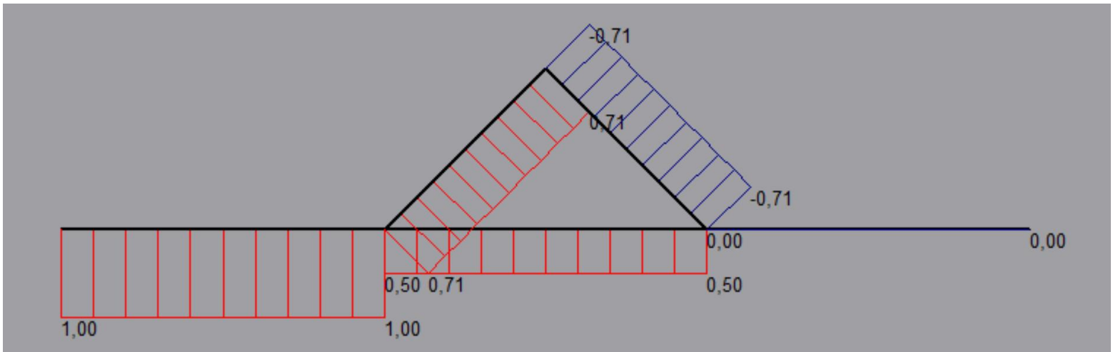
Διάγραμμα αξονικών
