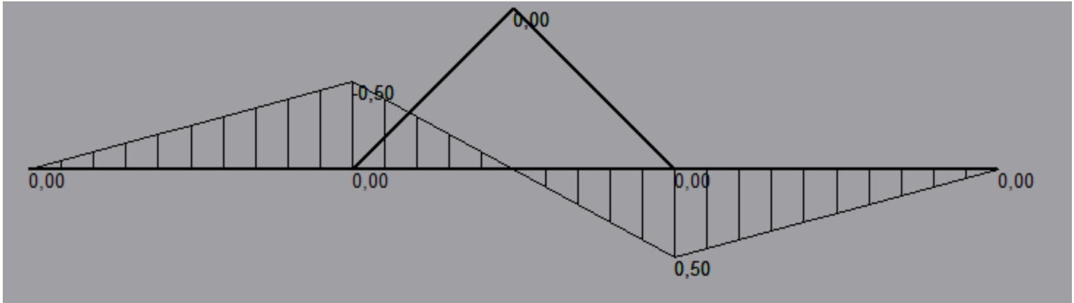
Διάγραμμα τεμνουσών
