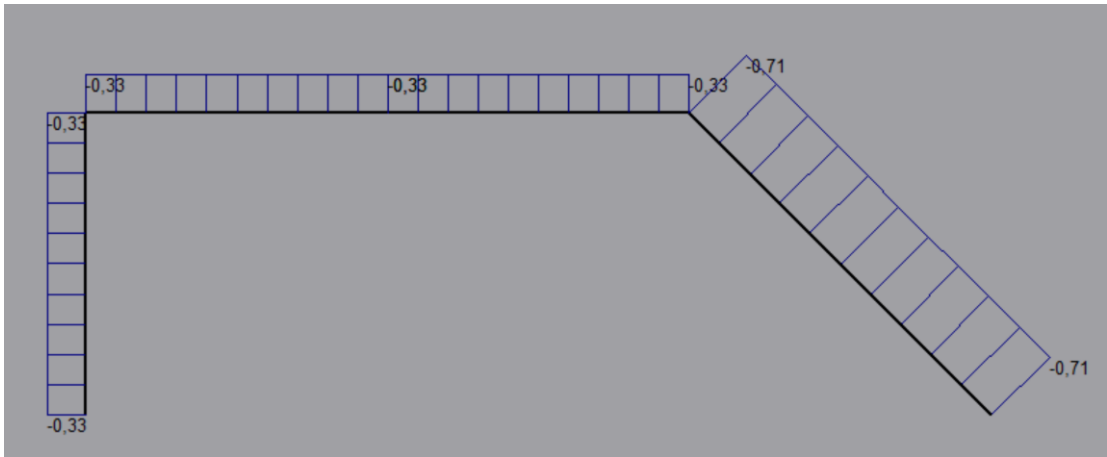
Διάγραμμα αξονικών
