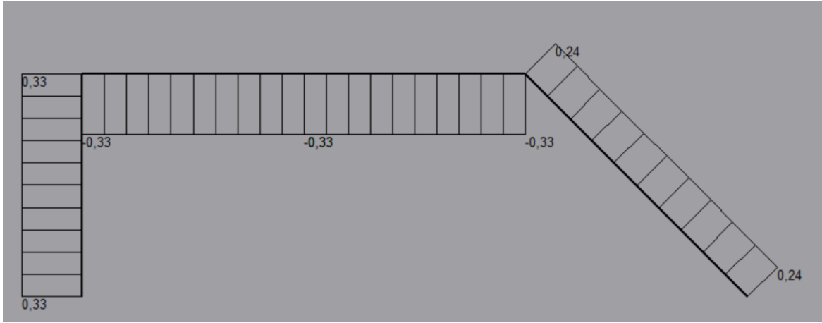
Διάγραμμα αξονικών
