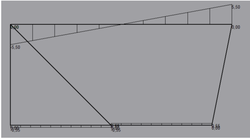
Διάγραμμα αξονικών
