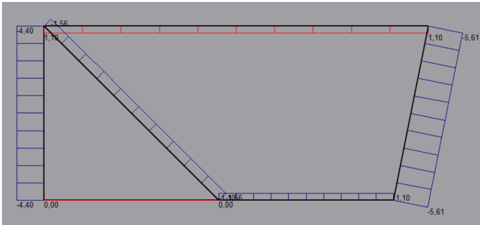
Διάγραμμα αξονικών
