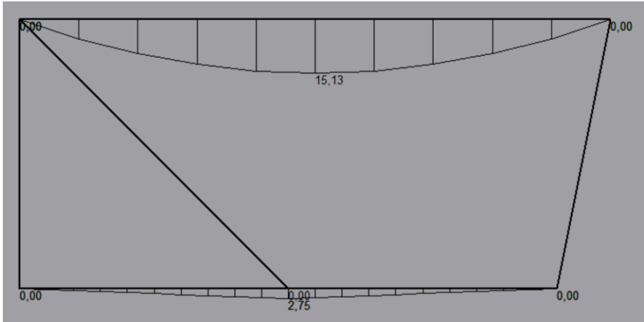
Διάγραμμα τεμνουσών
